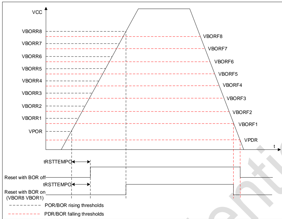
图 2-3 POR/PDR/BOR 阈值
