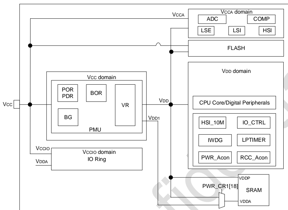
图 2-2 电源框图
